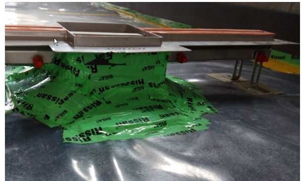
Die Abläufe der Rinnen wurden entkoppelt, die Füsse der Rinnen dürfen nicht verschraubt werden
