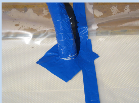
Leitungsdurchdringungen sauber abgepolstert und dicht verklebt.
