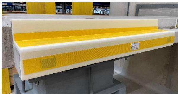
Abbildung 18: ISOTREPP® "28dB" TL-4000 Austritt (Z-Form)
