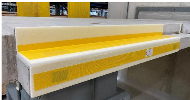
Abbildung 17: ISOTREPP® "28dB" TL-2000 Austritt (Z-Form)
