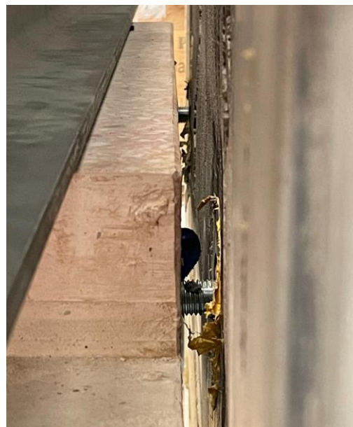
Abbildung 12: Luftfuge e = 20mm zwischen Podest und Wand: Gewindestangen M20, welche im Schallschutzgehäuse ISOSCALA®-43-10-IG aufgelagert sind
